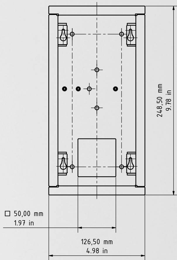
Unterputzgehäuse
